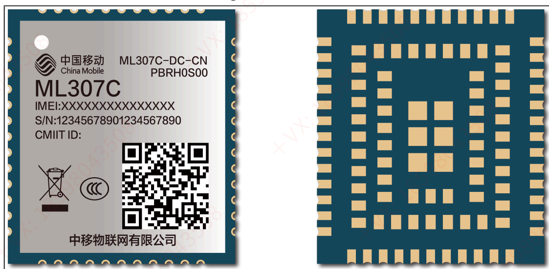
Figure 1. 模组示意图
