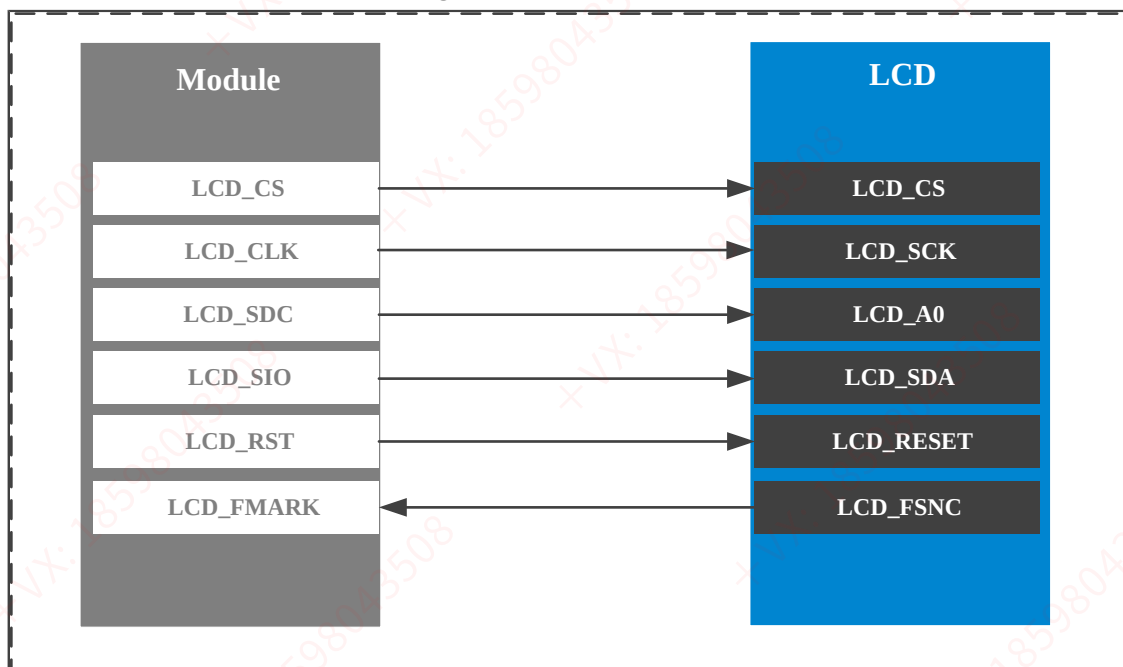
Figure 10. LCD接口示意图
