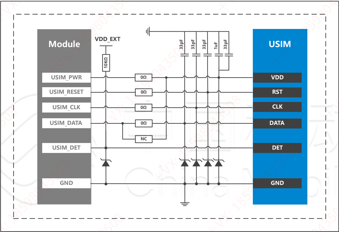
Figure 11. USIM接口示意图
