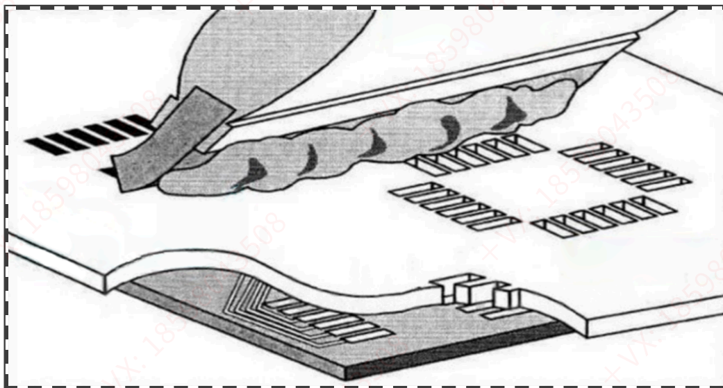
Figure 23. 印膏图
