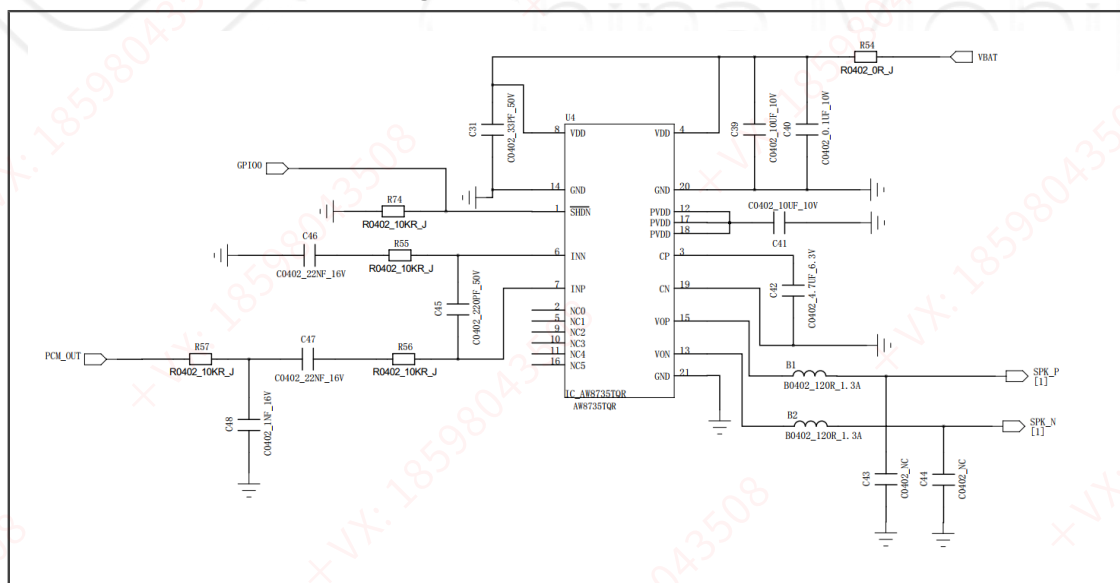
Figure 12. PWM方案参考设计
