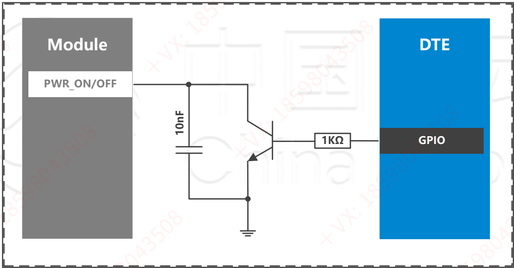
Figure 14. 模组开关机接口示意图
