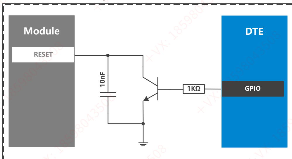
Figure 17. 模组复位接口示意图
