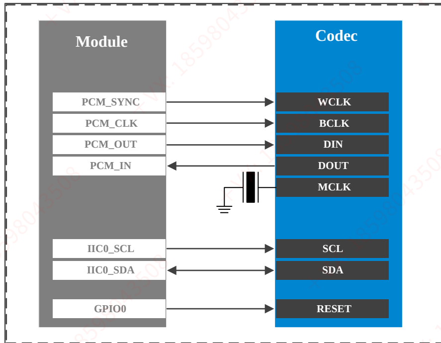
Figure 13. PCM接口示意图
