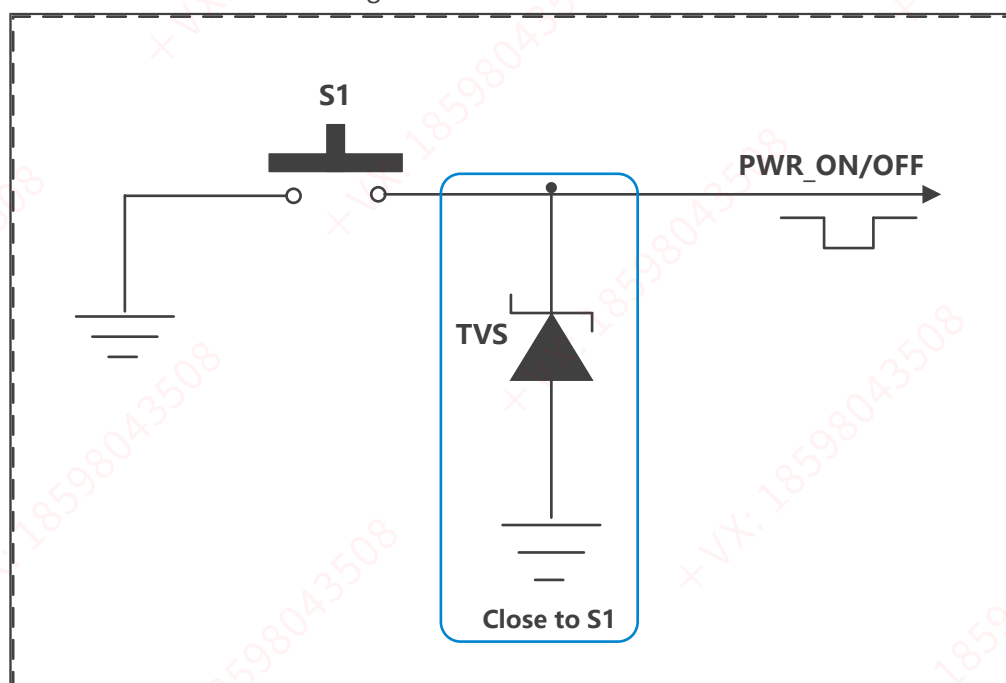
Figure 15. 开关机按钮示意图
