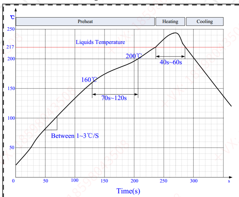
Figure 24. 炉温曲线
